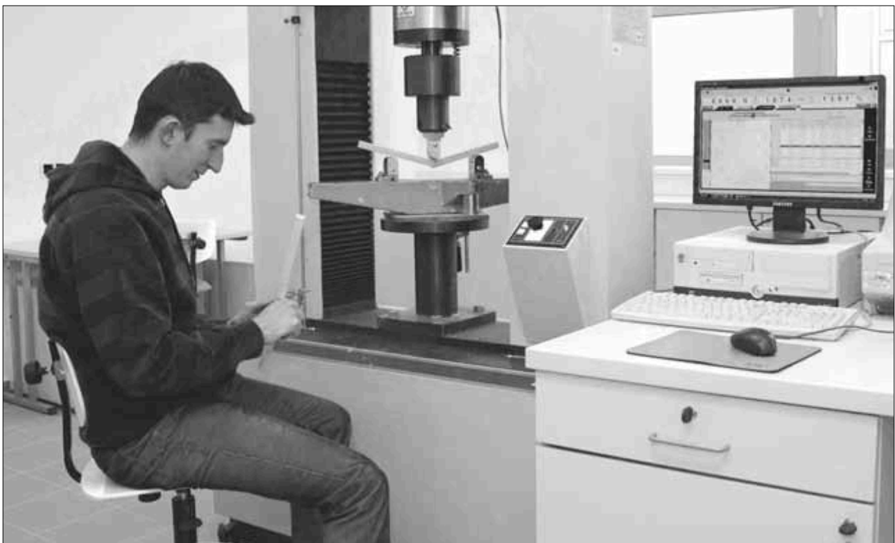
2. kép Faanyag mechanikai tulajdonságainak vizsgálata
