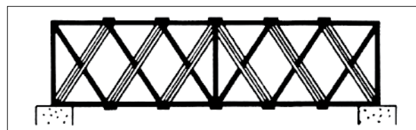
23. ábra A Brown-féle rácsos tartó kialakítása (Forrás: Raymond E. Wilson 1976)
