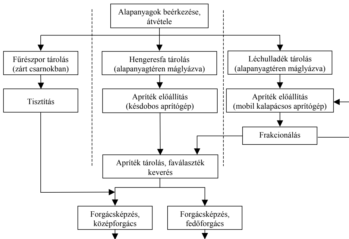
2. ábra – A vizsgált technológia folyamatábráj
