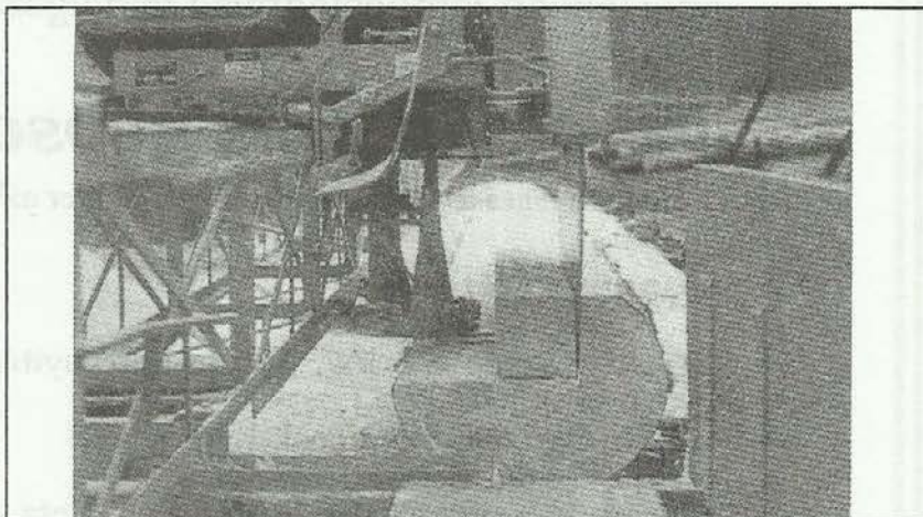
1. ábra. Mobil T.128 számú USA fűrészgép, nagyméretű rönk felvágása közben.
