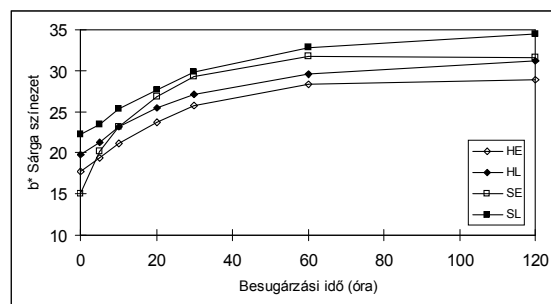
5. ábra – A japán ciprus pásztaí sárga színezetének változása napsugárzás hatására (Jelölések: H; geszt, S; szijács, E; korai pászta, L; késői pászta)
