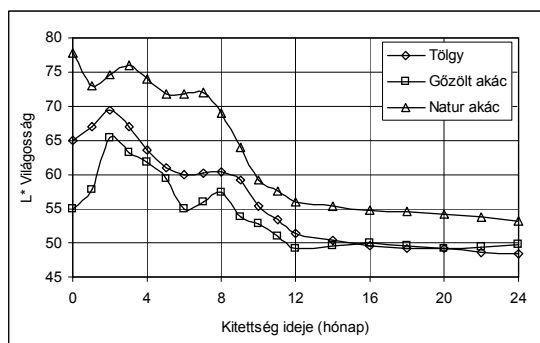
1. ábra – Az időjárás hatásának kitétt minták világosság-változásának időfüggése
