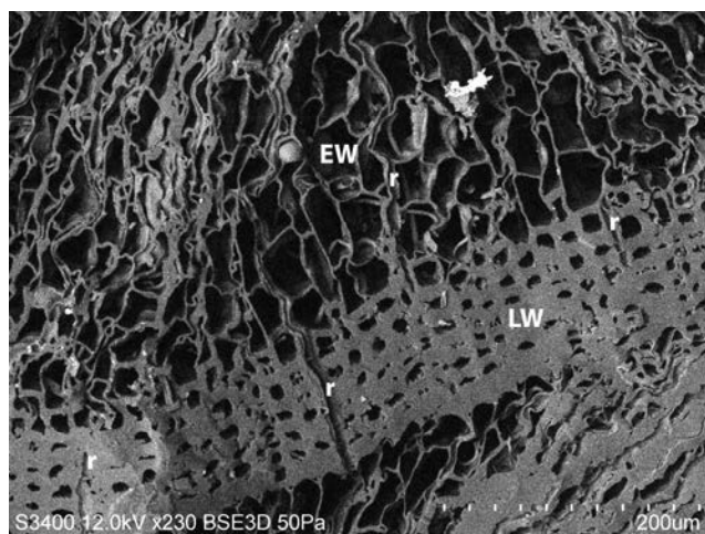
4. ábra – Az 5. minta keresztmetszetének SEM felvétele. Jól láthatók a korai pászta (EW) összenyomott tracheidái, a késői pászta (LW) vastagfalú tracheidái és néhány bélsugar. SEM, 230×
