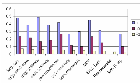
9. ábra – Az oszlopdiagram a \mu , \mu_0 , és Rz értékeinek sorrendjét mutatja – fafajtól függően, gumitömítéssel mérve, 0,0302 m 2 felület és -0,2 bar nyomásnak megfelelő terhelés mellett
