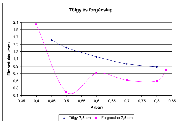
17. ábra – Tölgy és forgácslap minták elmozdulása
