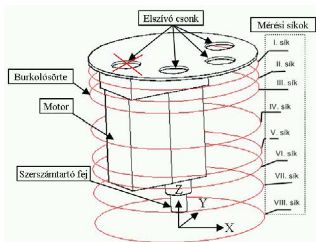
3. ábra. A mérési síkok elhelyezkedése
