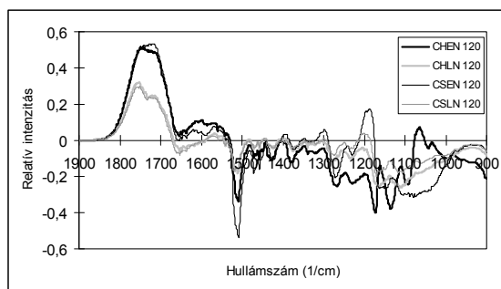
6. ábra – A japán ciprus pásztáinak infravörös, különbségi színeke 120 órás napsugárzás (N) hatására. (Jelölések: C; japán ciprus, H; geszt, S; szijács, E; korai pászta, L; késői pászta)
