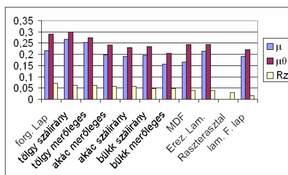
10. ábra – Az oszlopdiagram a \mu , \mu_0 , és Rz értékeinek sorrendjét mutatja – fafajtól függően, gumitömítés nélkül mérve, 0,0723 m 2 felület és -0,6 bar nyomásnak megfelelő terhelés mellett
