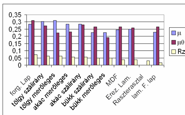
8. ábra – Az oszlopdiagram a \mu , \mu_0 , és Rz értékeinek sorrendjét mutatja – fafajtól függően, gumitömítéssel mérve, 0,0723 m 2 felület és -0,6 bar nyomásnak megfelelő terhelés mellett
