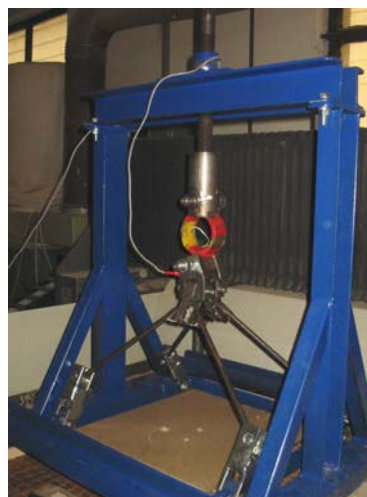
4. ábra – Munkadarab leszakító berendezés mérő gyűrűvel
