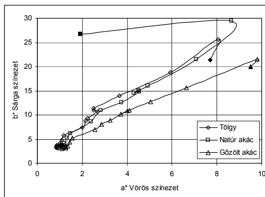
2.ábra – A színpontok vándorlása a kitétség hatására (A görbék fekete kezdőpontjai a kezeletlen minták színpontjai, és ezeket követik a havonta, a második évben kéthavonta mért színpontok.)
