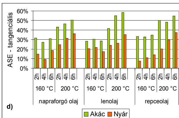
1. ábra – Az akác és a nyár nyomószilárdságának (a), hajlítószilárdságának (b), radiális zsugorodásának (c), tangenciális zsugorodásának (d), L^* (e), a^* (f), b^* (g) színkoordinátájának és színinger különbségének (h) változása az OHT (forró olajos kezelés) hatására
