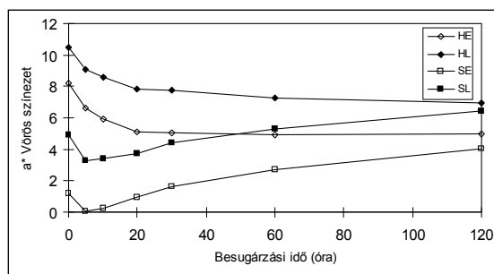
4. ábra – A japán ciprus pásztaí vörös színezetének változása napsugárzás hatására (Jelölések: H; geszt, S; szijács, E; korai pászta, L; késői pászta)
