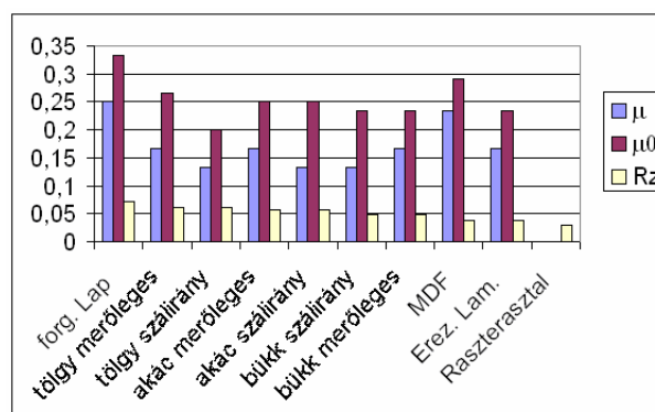
11. ábra – Az oszlopdiagram a \mu , \mu_0 , és Rz értékeinek sorrendjét mutatja – fafajtól függően, gumitömítés nélkül mérve, 0,0302 m 2 felület és -0,2 bar nyomásnak megfelelő terhelés mellett
