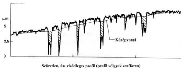
5. ábra – Születlen, úgynevezett elsődleges 'P' profil
