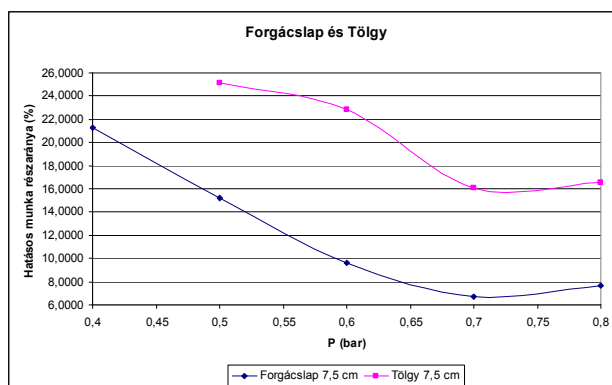
16. ábra – Forgácslapnál és tölgynél a hatásos munka részaránya
