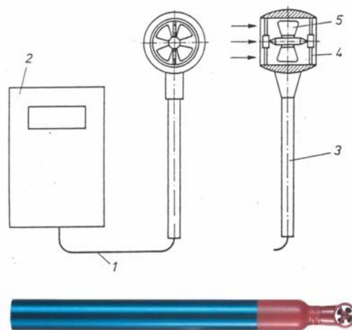
2. ábra – Szárnylapátos anemométer 1) összekötő kábel; 2) kijelző műszer és áramforrás; 3) fogantyú; 4) függesztőborda; 5) járókerék
