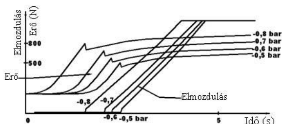
2. ábra – Erő és elmozdulás regisztrátum forgácslapnál
