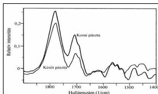
7. ábra – Az éger szijácsa korai és késői pásztájának infravörös, különbségi színeke 30 órás xenonlámpás besugárzás esetén
